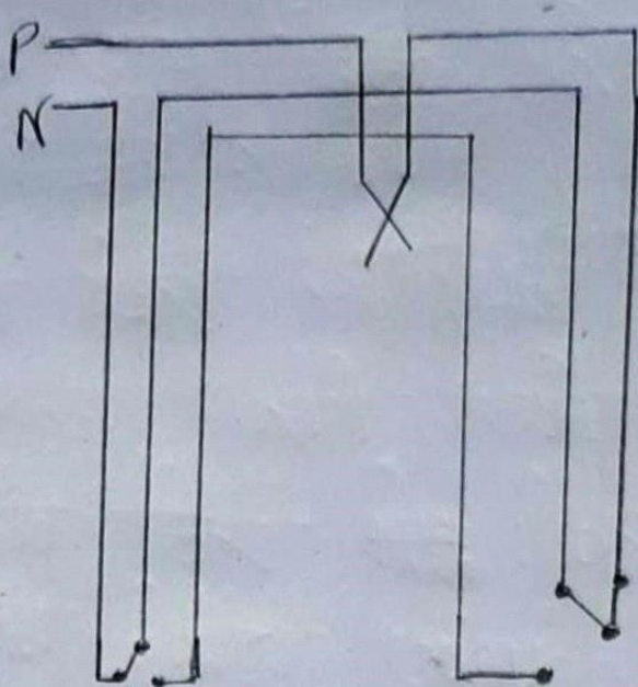
(मल्टीलाइन वायरिंग)
