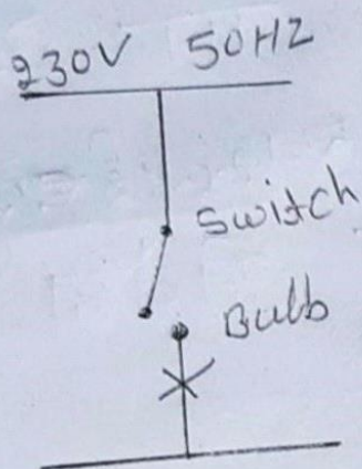
(सिंगल बिन्दु चित्र)
