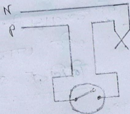
(मल्टी लाइन वायरिंग)
